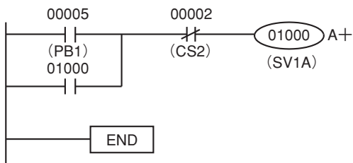
図 5-9 自己保持回路
